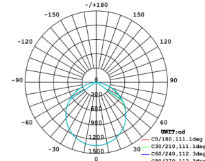
60x60 fénygörbe
