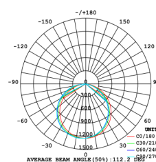
30x120 fénygörbe
